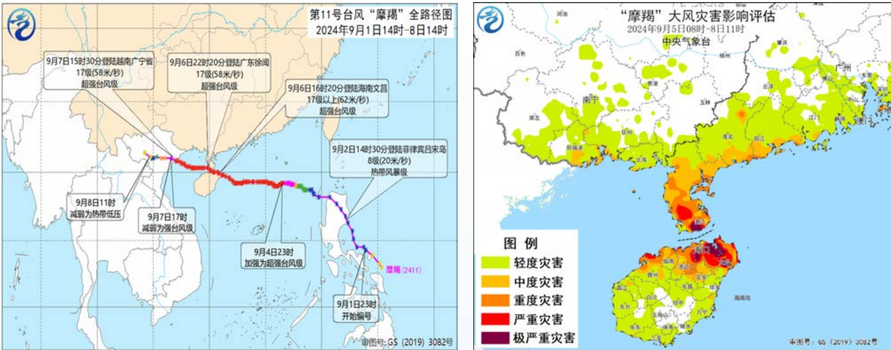
图 1.6 2024 年第 11 号台风“摩羯”路径（左）和大风灾害影响评估（右）
